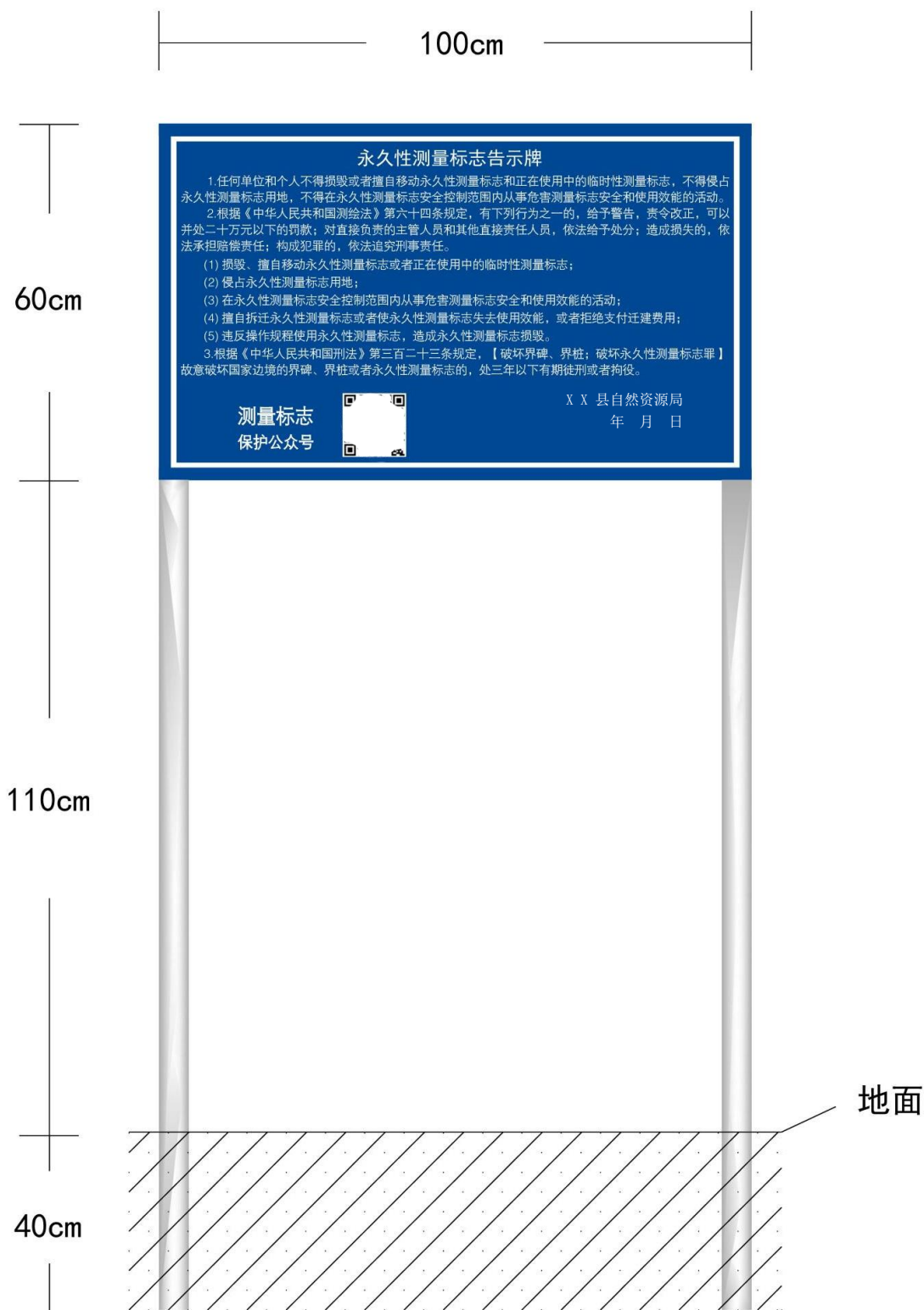
图 2 测量标志保护标识牌背面
