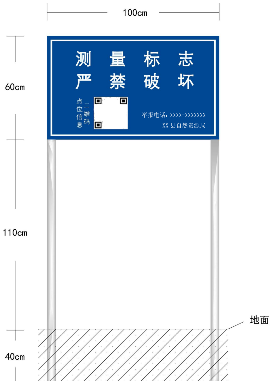
图 1 测量标志保护标识牌正面
